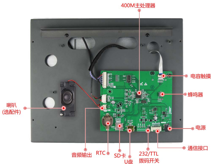
图 1-2 硬件配置图
