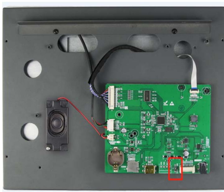
图 8-2 电平转换开关位
